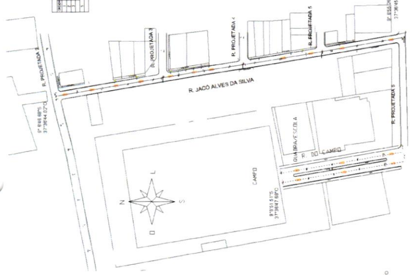
PLANTA DE DRENAGEM SUPERFICIAL BAIRRO TANCREDO NEVES ESC. 1:500
