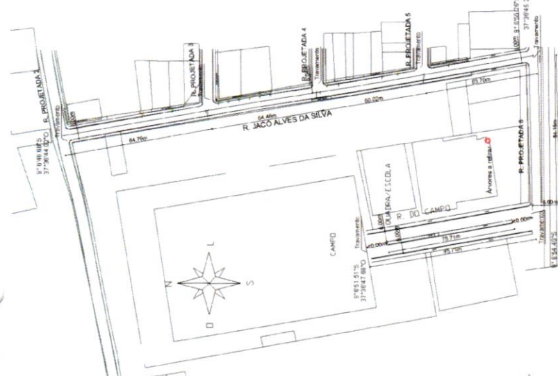
PLANTA DE COTAS BAIRRO TANCREDO NEVES ESC. 1:500
